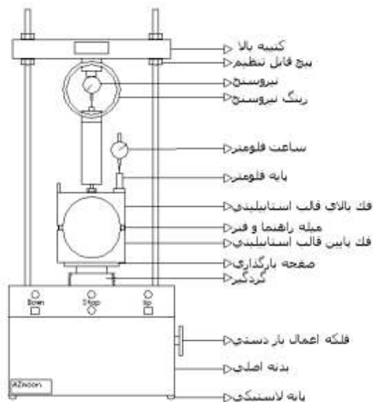
شکل شماتیک جک مارشال
